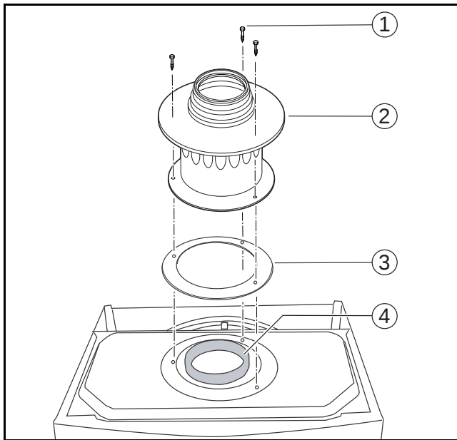
Res. 12 B 22 Tipi Atık Gaz Tahliyesi
