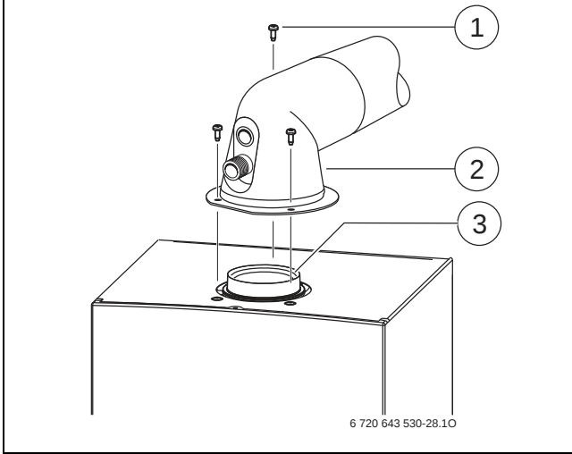
Res. 11 Atık Gaz Tahliye Aks. Montajı
