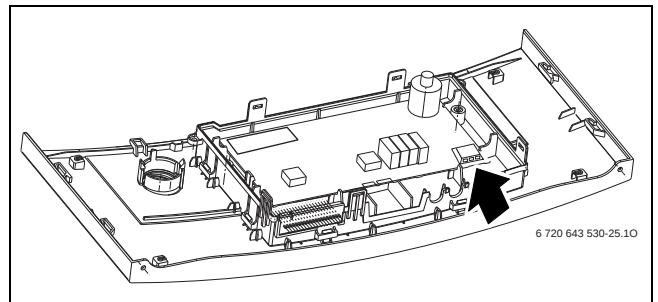
Res. 17 230 VAC Şebeke Kablosu Bağlantısı
