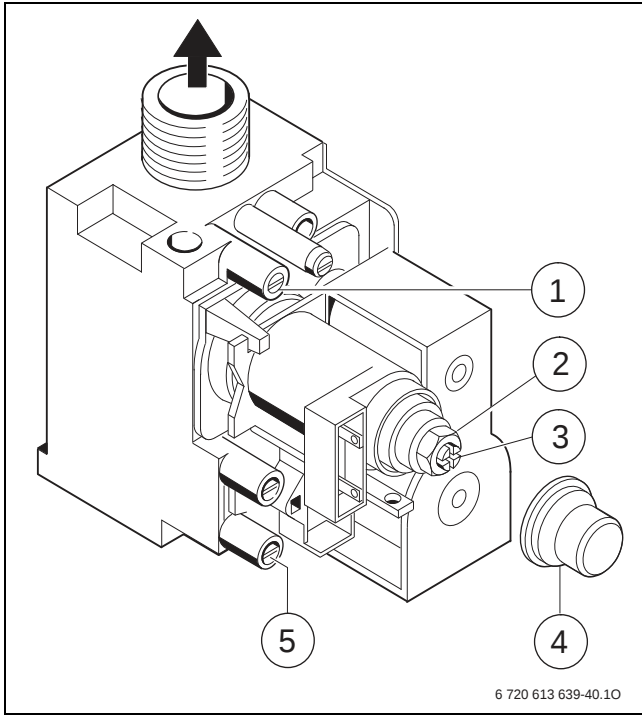
Res. 31 Gaz Armatürü
